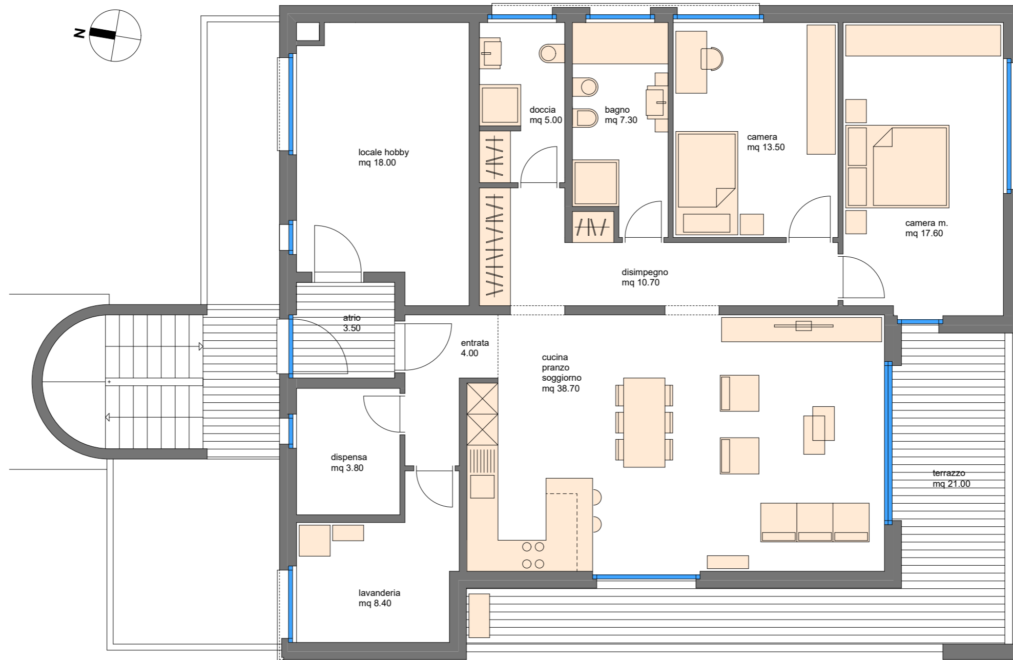
PIANTA SECONDO PIANO
